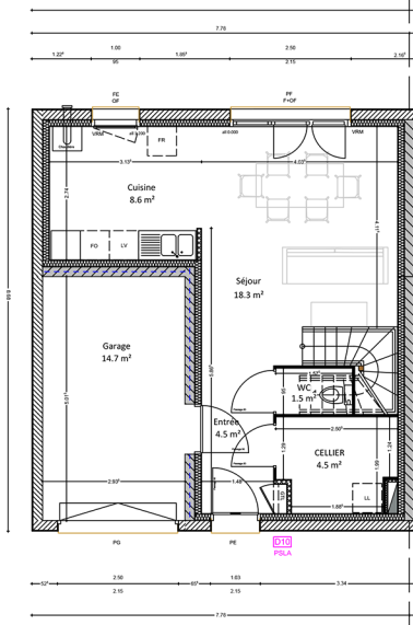
PLAN RDC
